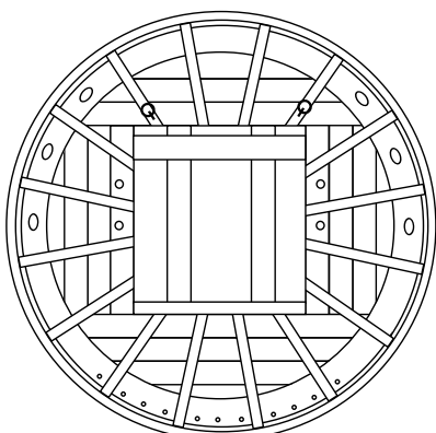
Großmars
